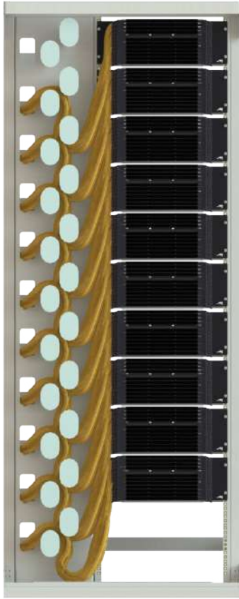
FIGURA 2. Gabinete interior de alta densidad (Organizador izquierdo) completamente ruteado. Con distribuidores FD -4UHD con acopladores LC*
