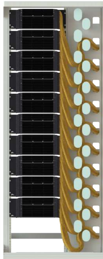
FIGURA 3. Gabinete interior de alta densidad (Organizador derecho) completamente ruteado. Con distribuidores FD -4UHD con acopladores LC*
