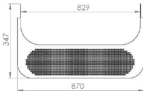
FIGURA 8. VISTA SUPERIOR
