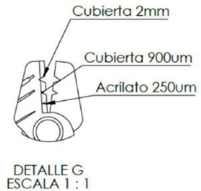
Fig 4: Cuchillas de desforre
