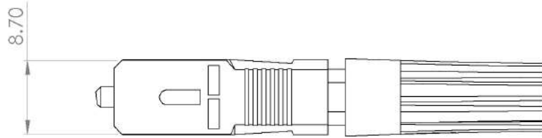
Fig. 3 Vista posterior del conector
