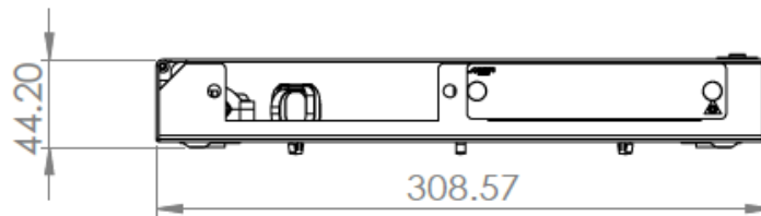
Fig. 2 Vista frontal
