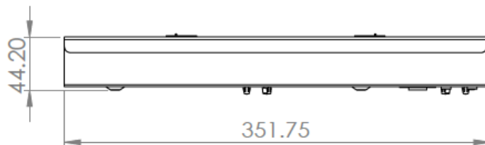
Fig. 3 Vista lateral
