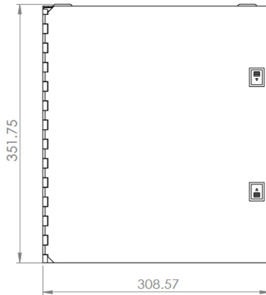
Fig. 1 Vista superior
